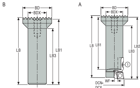
1. Śruba montażowa
