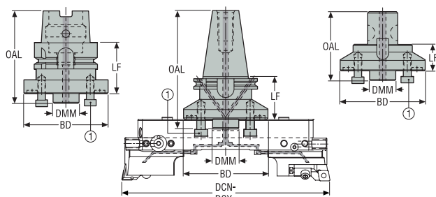
1. Śruba regulacyjna
