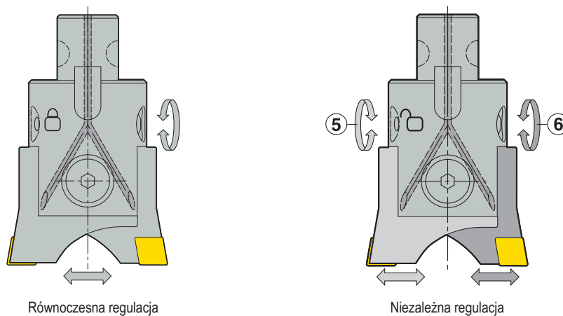
Równoczesna regulacja
